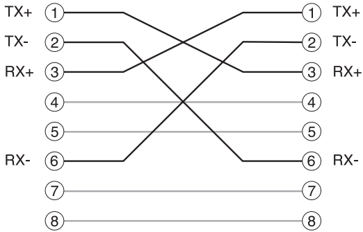
Cat5e Crossover Wiring
