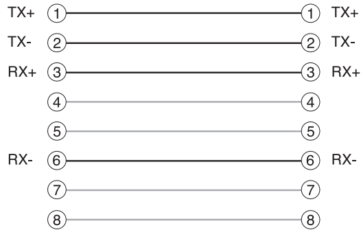
Cat5e Straight Wiring
